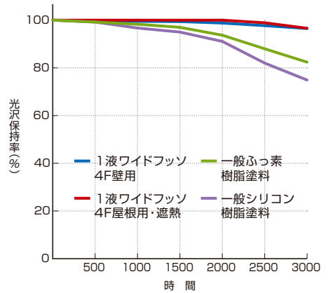
促進耐候性試験結果(キセノンランプ法)
