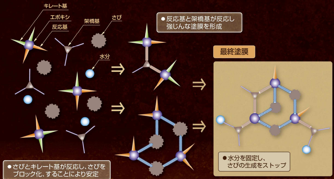
さびストップの防さび機構(例)
